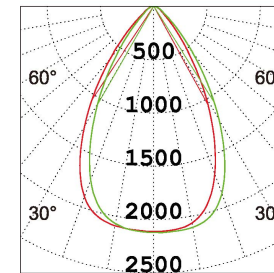
3×10W 3000K 60 °
