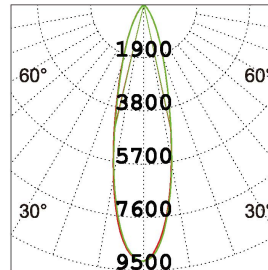
2×15W 3000K 24 °
