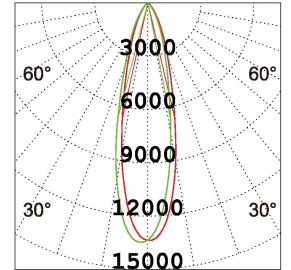
3×15W 3000K 24 °
