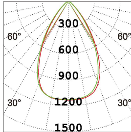
15W 3000K 60 °
