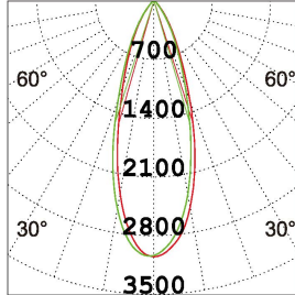
15W 3000K 36 °
