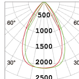
3×10W 3000K 60 °
