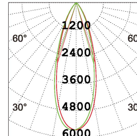
3×10W 3000K 36 °
