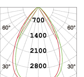
3×15W 3000K 60 °
