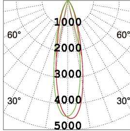
15W 3000K 24 °
