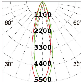
2×10W 3000K 24 °
