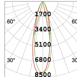
3×10W 3000K 24 °
