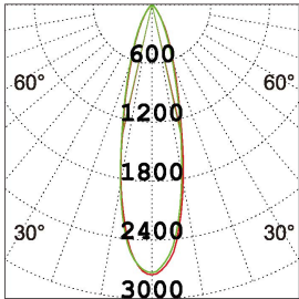
10W 3000K 24 °
