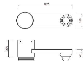
CCTV
